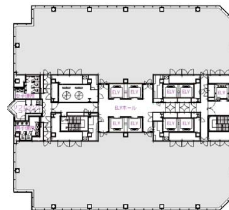
A棟基準階平面図（1フロア976㎡）
